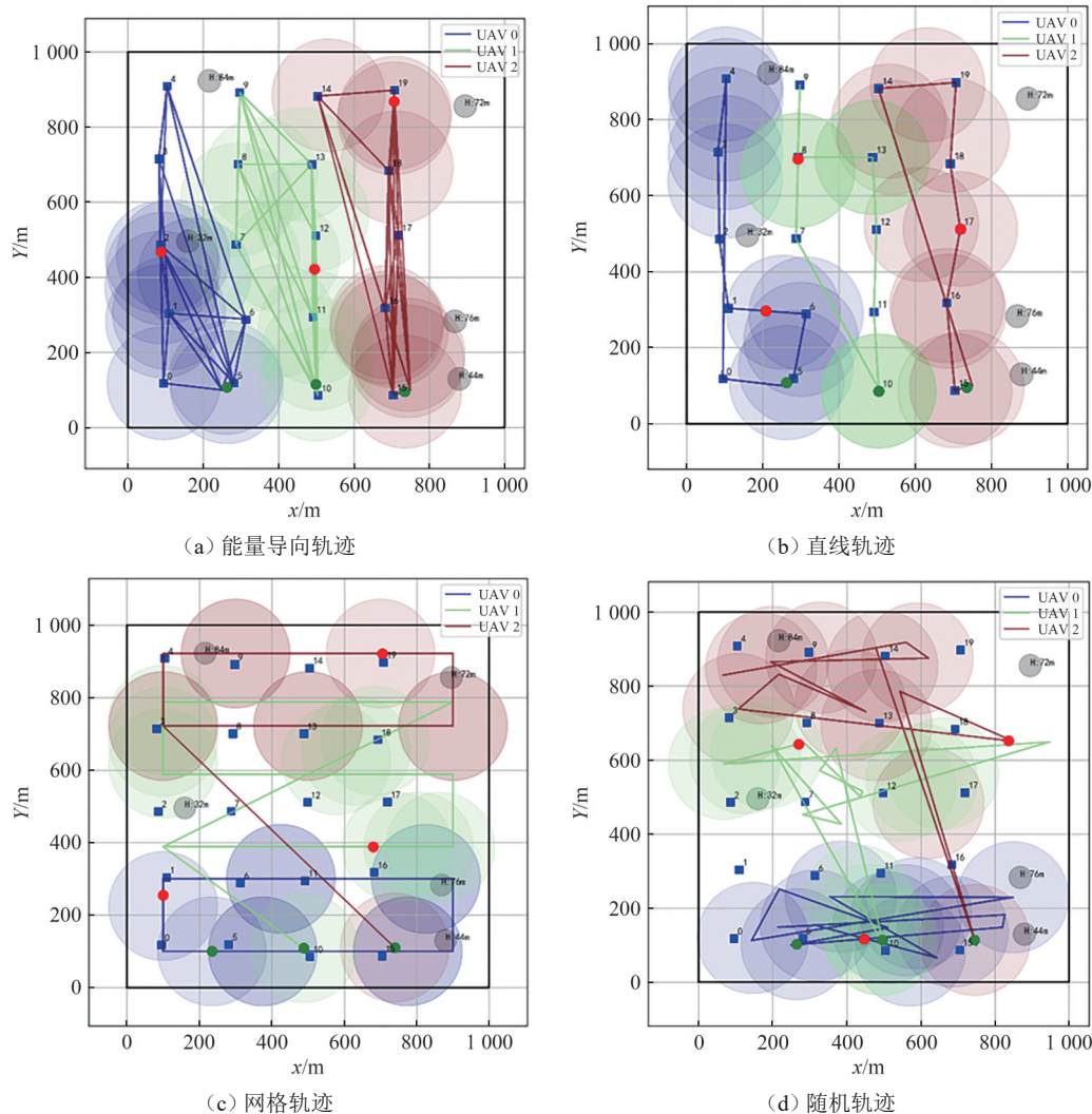
图3 不同轨迹规划算法的UAV运动轨迹示例
