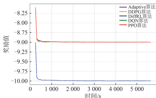
图5 不同算法收敛性对比
