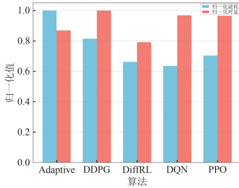
图8 各算法归一化能耗与时延对比
