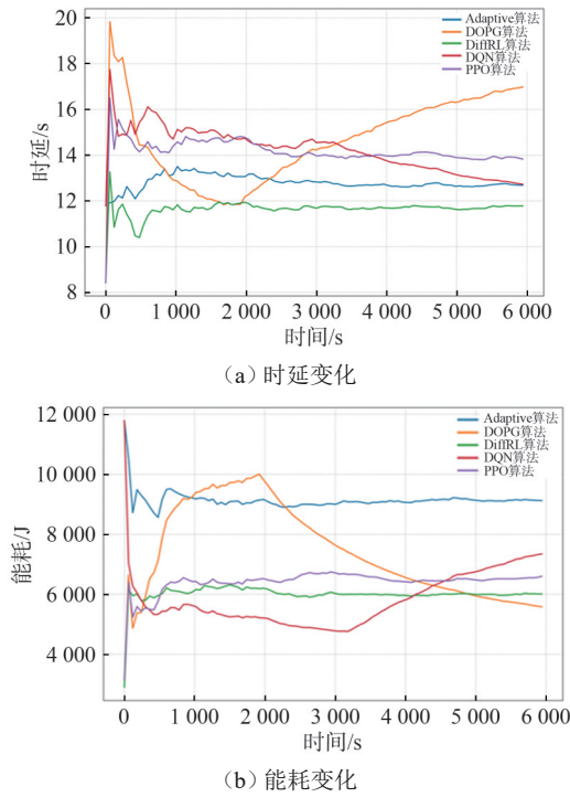
图7 不同卸载决策算法性能对比
