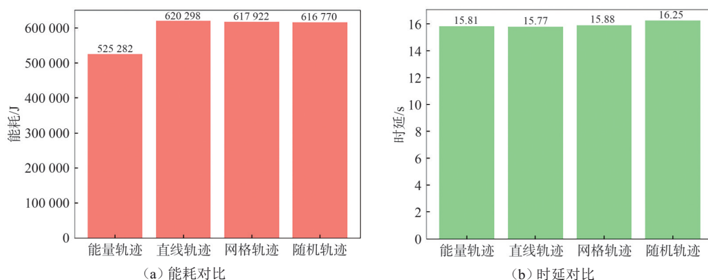
图2 不同轨迹规划算法的性能对比
